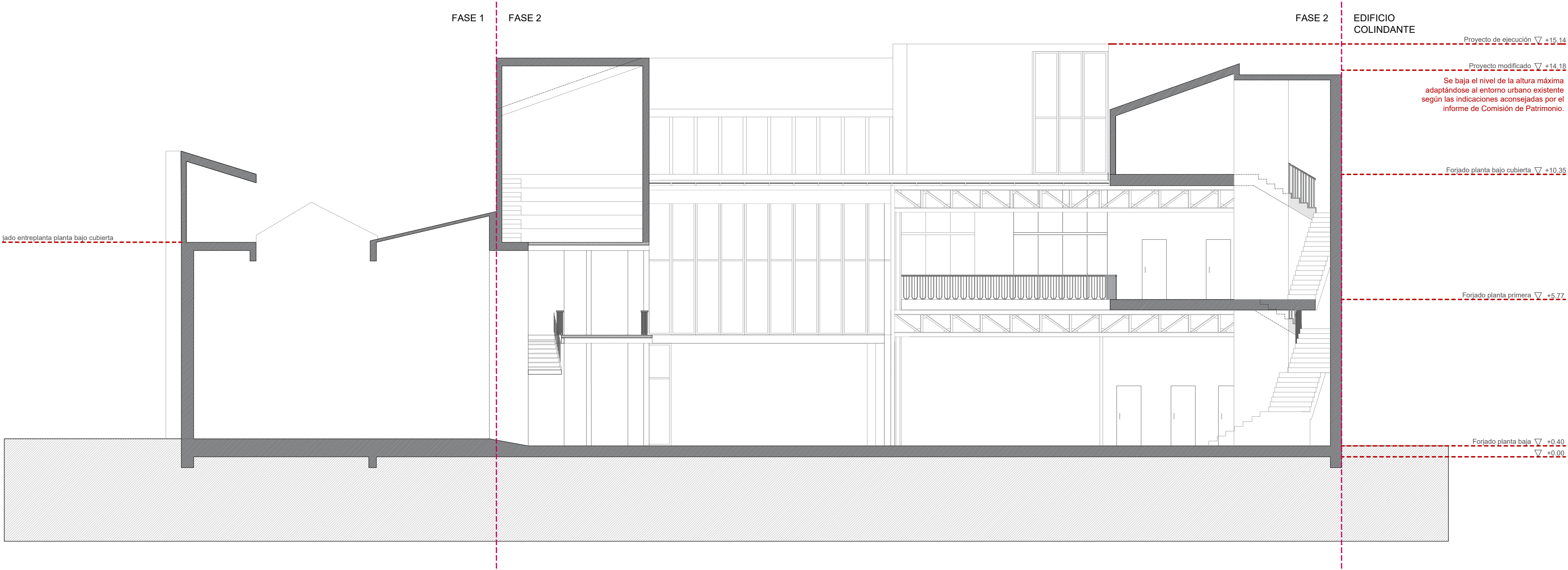
> SECCIÓN. PROYECTO DE EJECUCIÓN. Plaza de los Mártires_ e: 1/100
