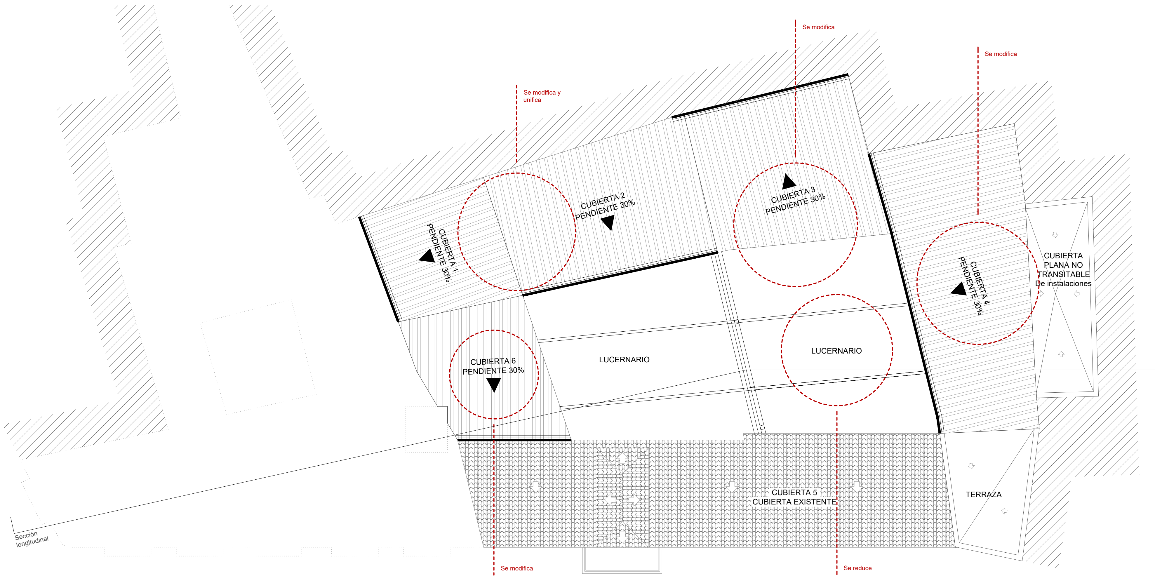
> PLANTA CUBIERTA. PROYECTO DE EJECUCIÓN. Plaza de los Mártires_ e: 1/100
