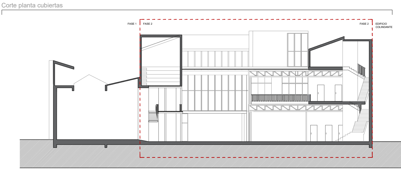
> SECCIÓN. PROYECTO DE EJECUCIÓN_ e: 1/300
