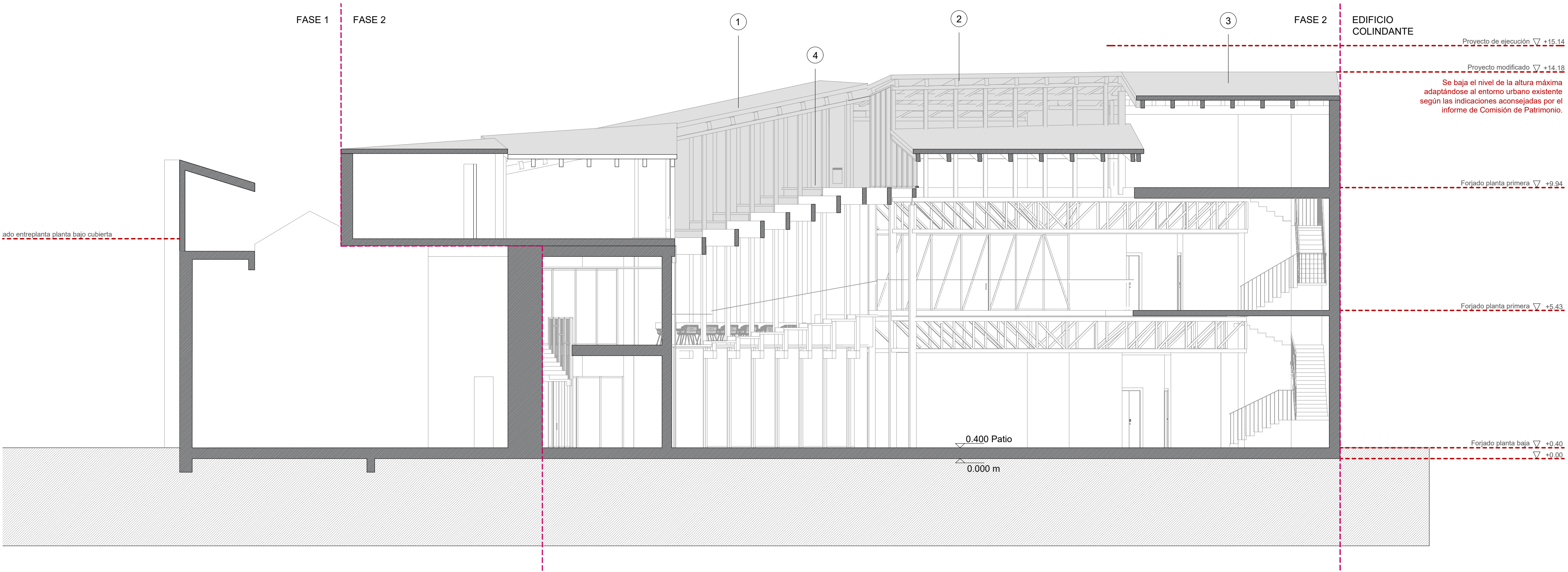
> SECCIÓN. MODIFICADO NOVIEMBRE 2022. Plaza de los Mártires_ e: 1/100
