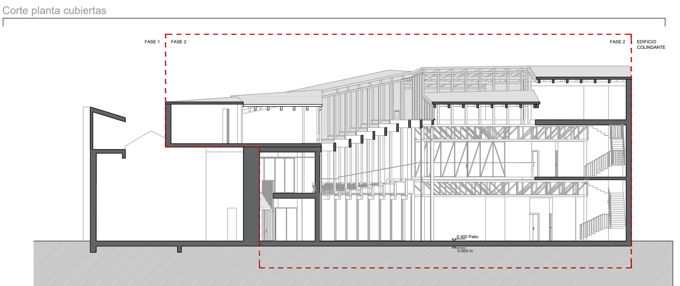
> SECCIÓN. MODIFICADO NOVIEMBRE 2022_ e: 1/300
